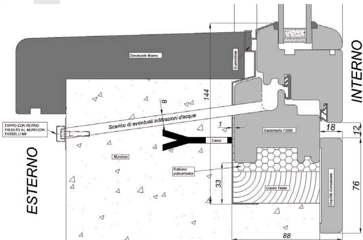
PARTICOLARE NODO INFERIORE
