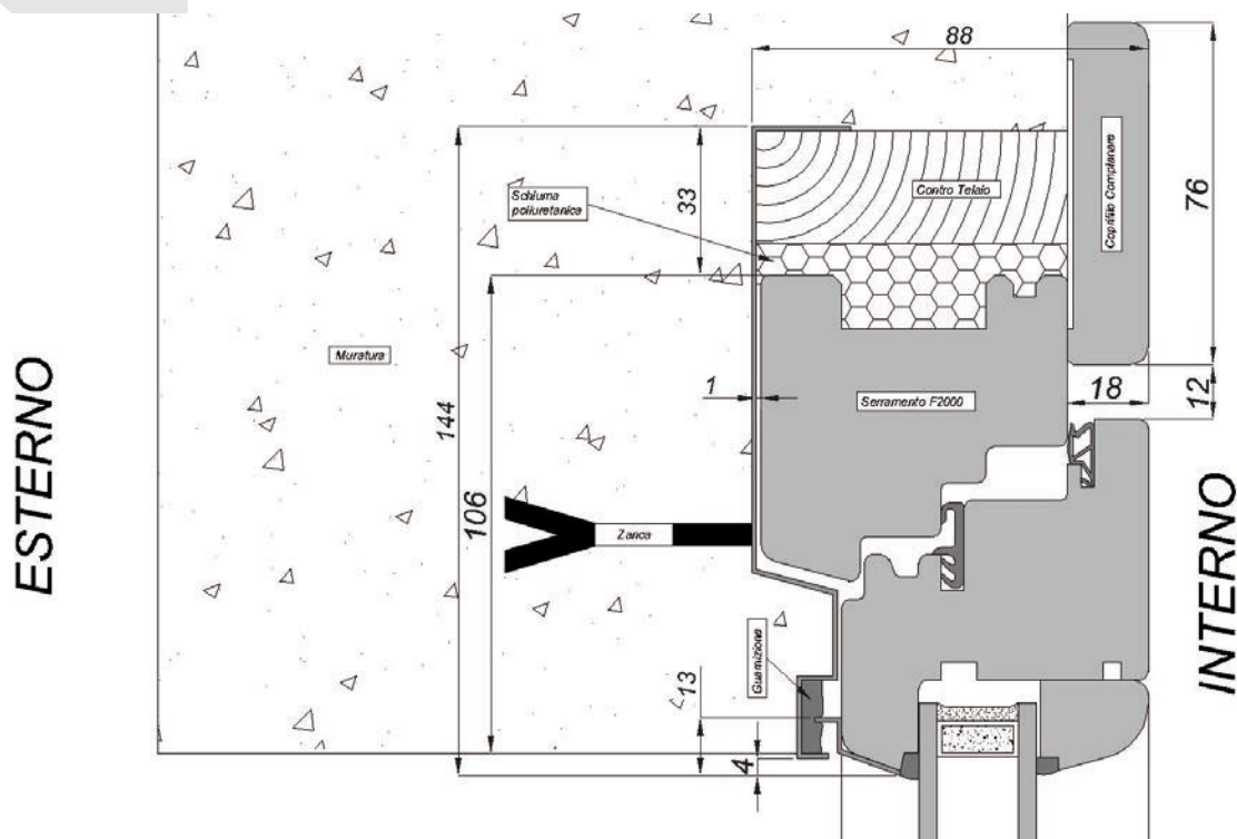
PARTICOLARE NODO SUPERIORE
